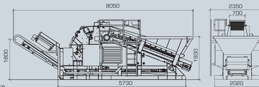
Position de service (données en millimètres)
